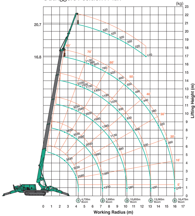
Outriggers Position : Max
