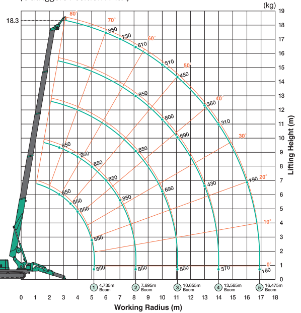
850kg Searcher Hook Offset Position : SH2 (Outriggers Position : Max)
